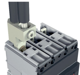
Ekstern FCCuAl tilkobling for kopper-/aluminiumskabler
